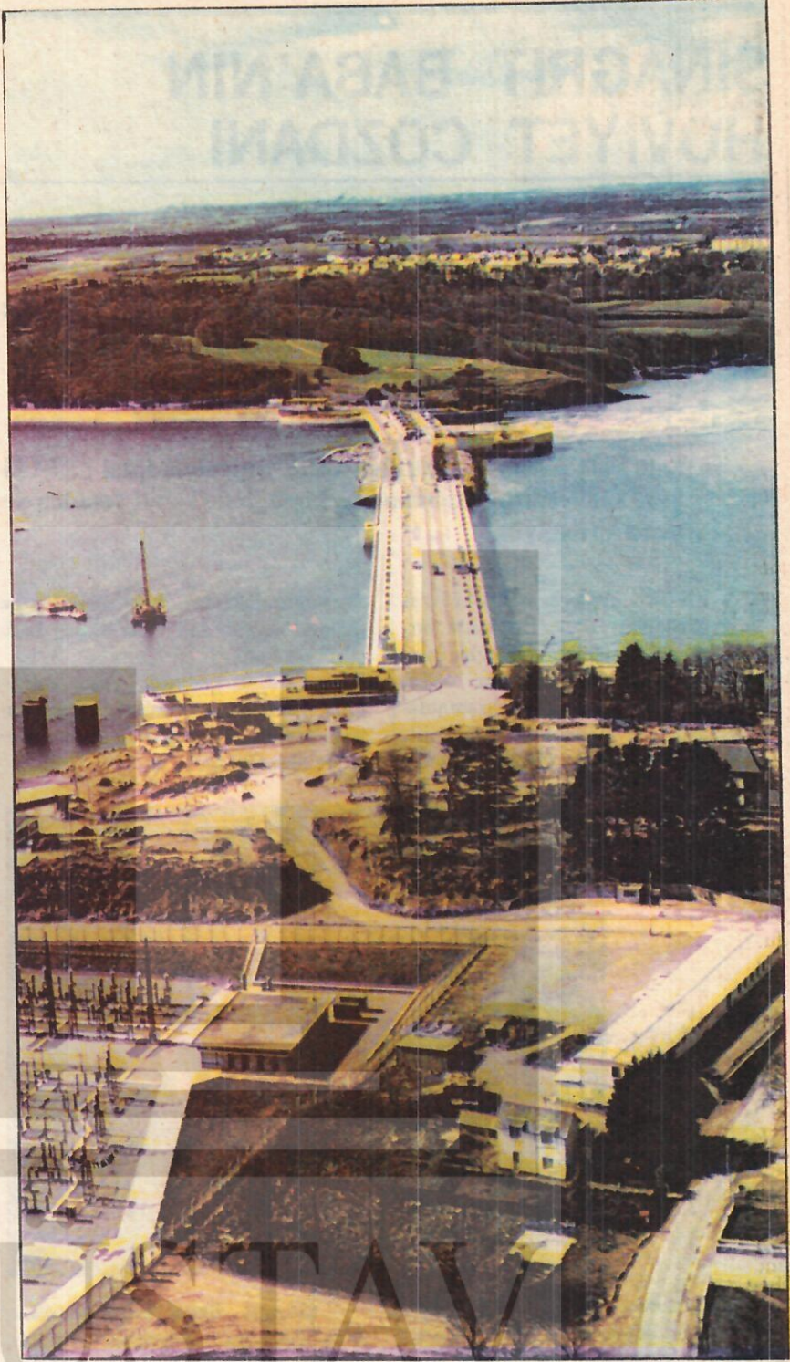
Yeni kaynak arayışı. Manş Denizi ağzında Rance gel-git santrali.
